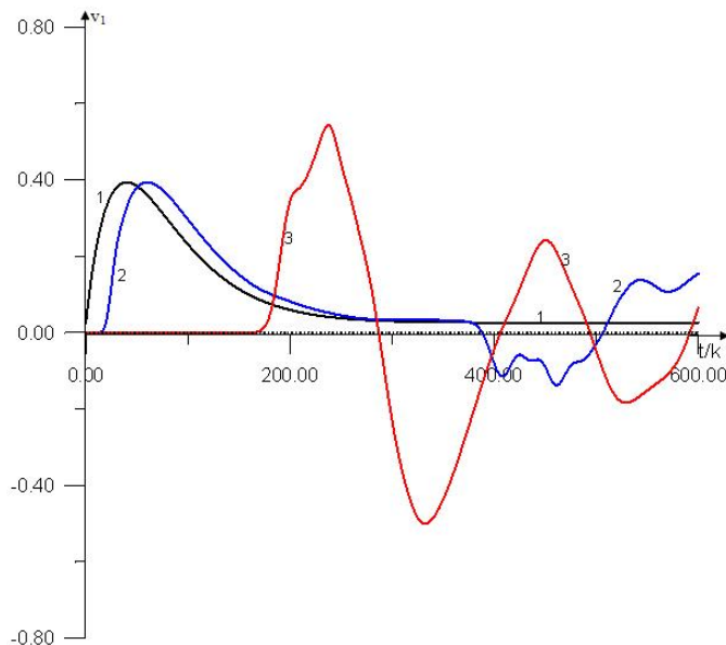
1 — точка (0, 0); 2 — точка (10, 25); 3 — точка (90, 25) Рисунок 4. Оциллограмма продольных скоростей перемещений v_1 в трех фиксированных точках наблюдения прямоугольной области
