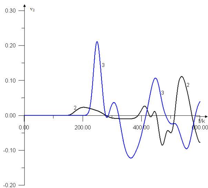
1 — точка (0, 0); 2 — точка (10, 25); 3 — точка (90, 25) Рисунок 5. Оциллограмма поперечных скоростей перемещений v_2 в трех фиксированных точках наблюдения прямоугольной области
